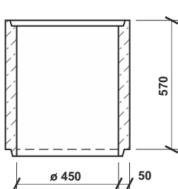
SKRUŽ STŘEDOVÁ TBV - Q 450 / 570 / 6d hmotnost: 110 kg
