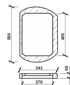
VYROVNÁVACÍ PRSTENEC TBV - Q 390 / 60 / 10b hmotnost: 9 kg
