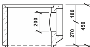
SKRUŽ HORNÍ TBV - Q 450 / 195 / 5c hmotnost: 40 kg
