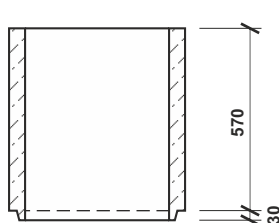
SKRUŽ HORNÍ TBV - Q 450 / 570 / 5d hmotnost: 110 kg
